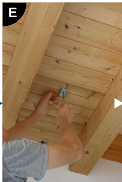
Stringere bene e verificare tenuta
