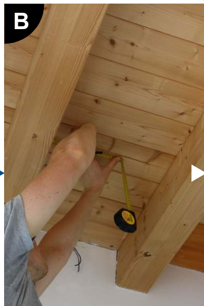
Misura per allineamento
